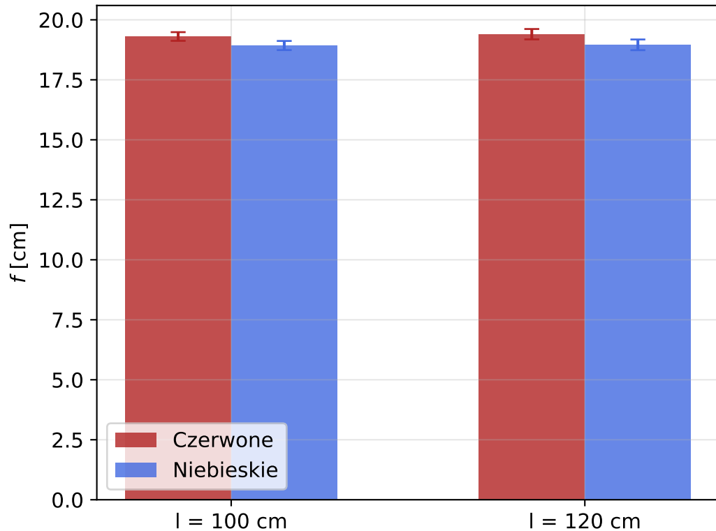
Ogniskowe – aberracja chromatyczna
