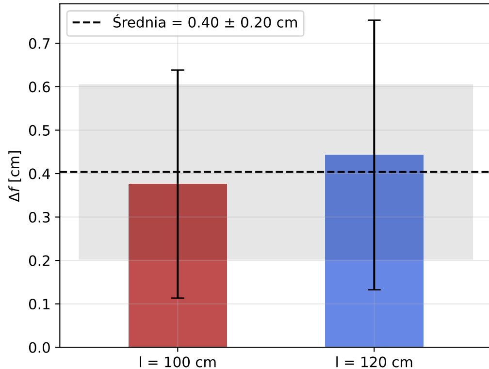
Aberracja chromatyczna \Delta f = f_{\text{czerw.}} - f_{\text{nieb.}}
